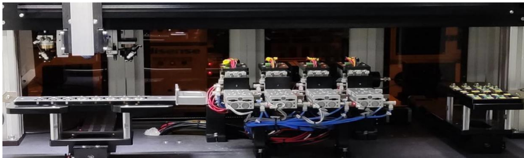
系统架构，并行4个测试载台
