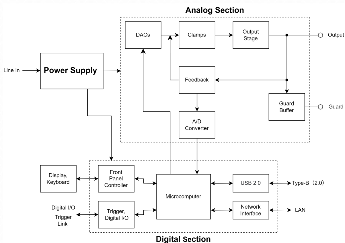
S3012H 架构图
